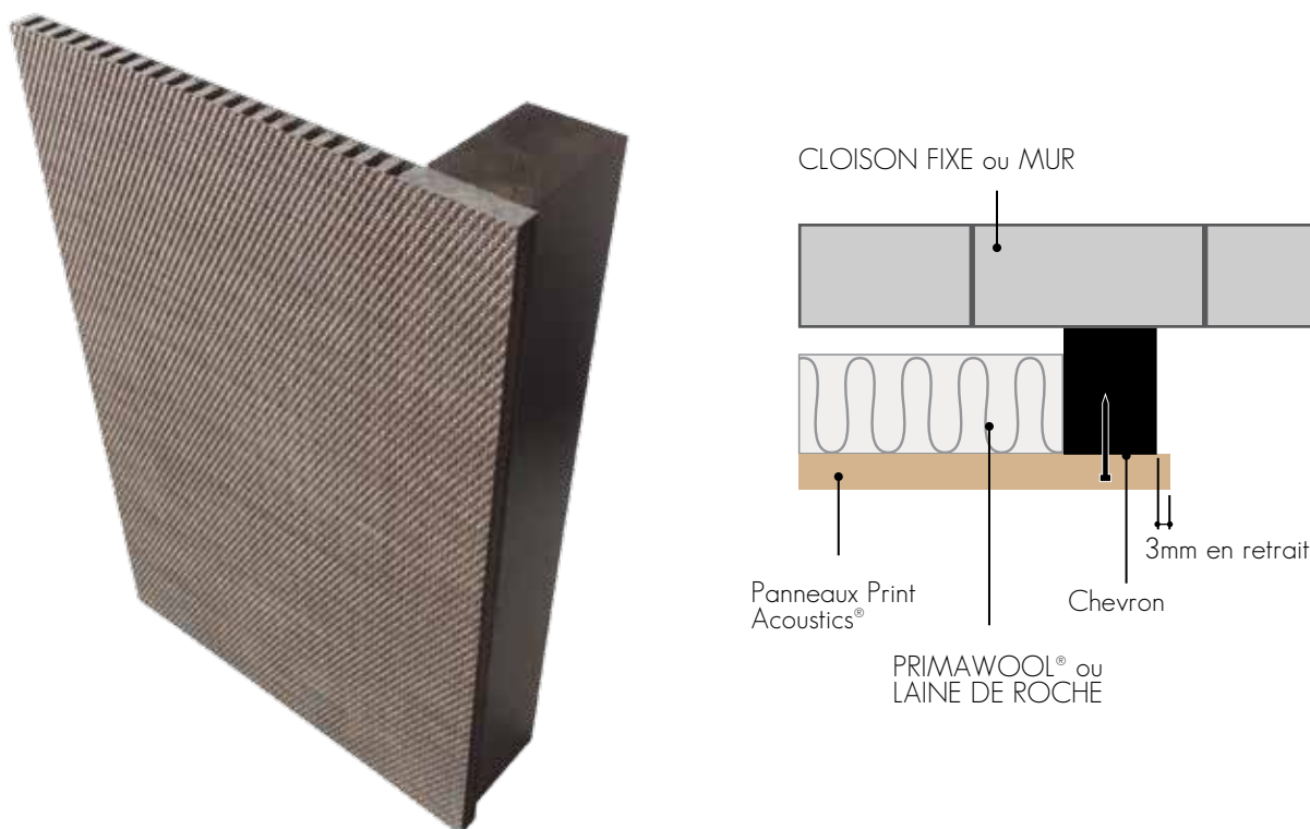
fig 22. Exemple avec chevron peint en retrait - TYPE I
