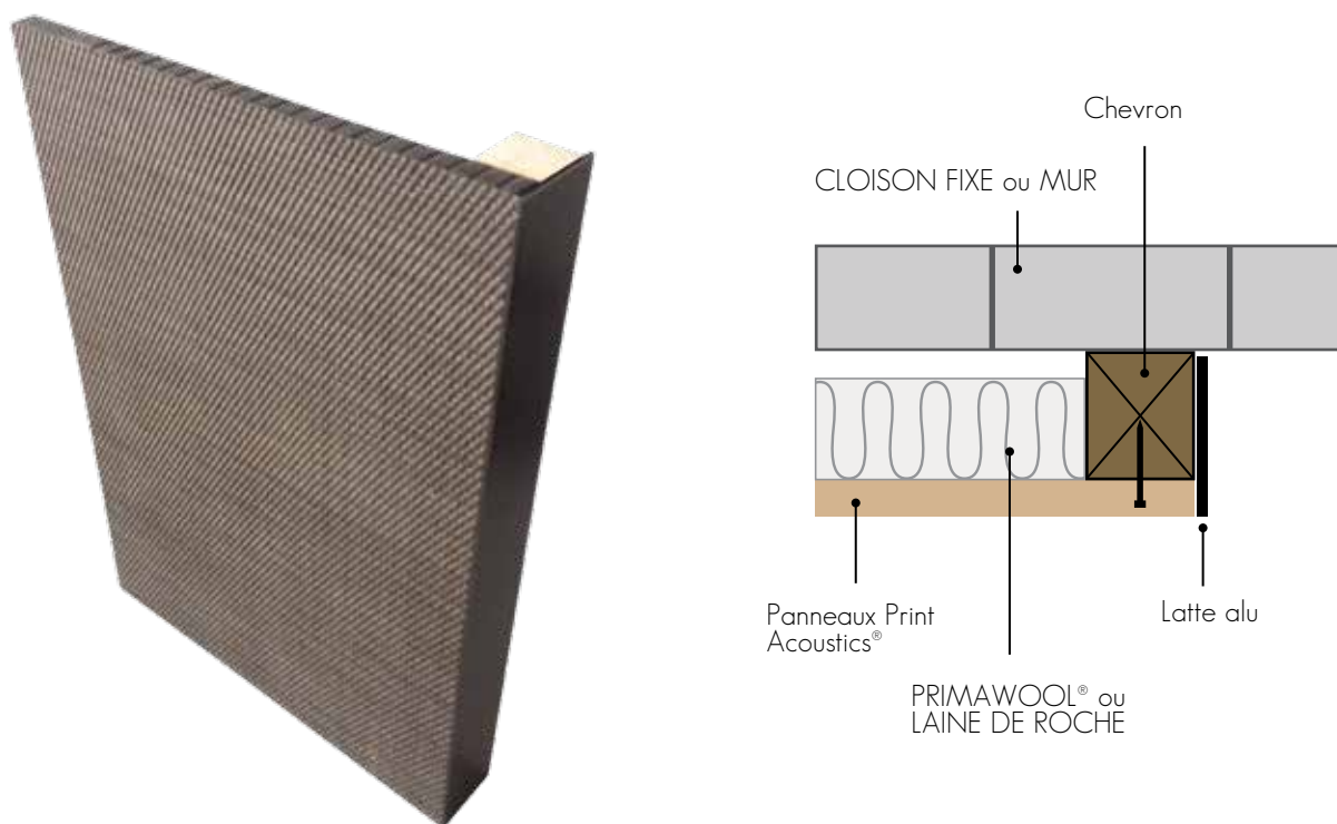
fig 21. Exemple avec latte alu - TYPE I
